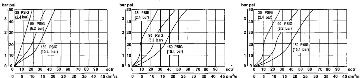
6 pav. Trijų tepalinių srauto charakteristikų pavyzdžiai.
