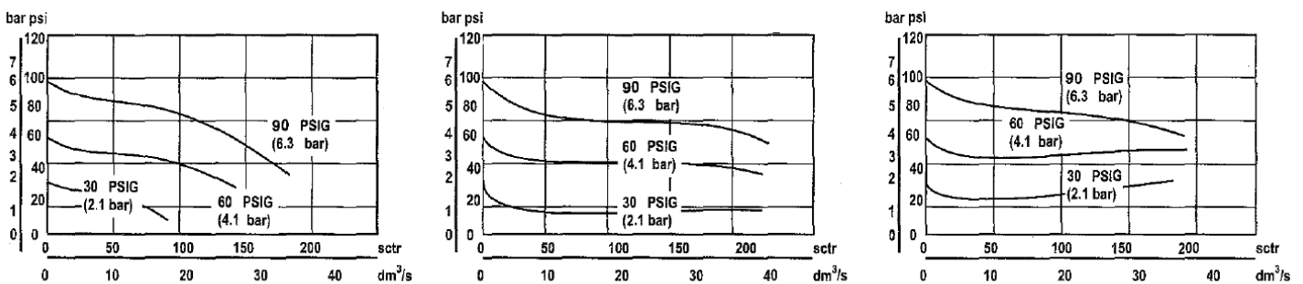
5 pav. Trijų slėgio sumažinimo vožtuvų srauto charakteristikų pavyzdžiai.
